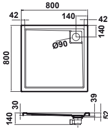
PLATO SIGMA CUADRADO 80x80 80x80 SQUARE SHOWER TRAY SIGMA
