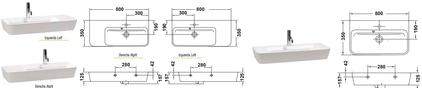
LAVABO ASIMÉTRICO COMPACT DE 80 cm. (mano derecha) # 27040 (mano izquierda) # 27045 80 cm. ASYMMETRICAL COMPACT WASHBASIN (right hand and left hand)
