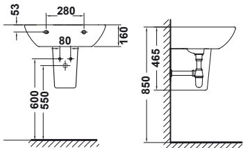
SEMICOLUMNA # 25432 OPCIÓN : LAVABO DE 55 # 25050 (REDONDO) / LAVABO DE 60 # 25040 (REDONDO) # 25030 (CUADRADO) SEMI-PEDESTAL
